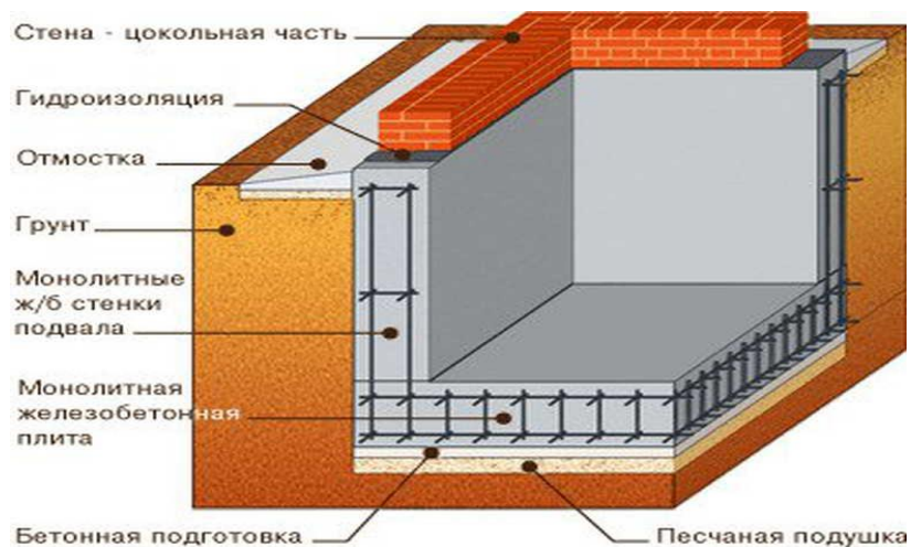
2-расм. Замонавий биоларнинг курсиси нам ўтказмаслик хусусиятига эга бўлган ва пойдевор конструкциясини арматура деталлари билан қучайтирилган курсининг ечими.
