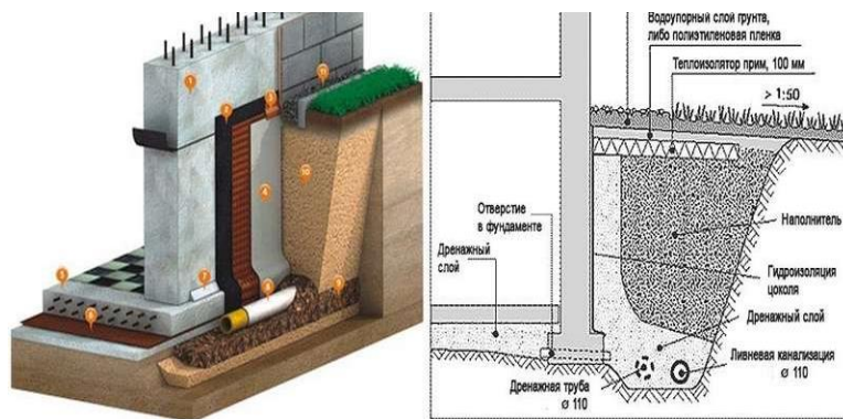
1-расм. Замонавий биноларнинг курсиси нам ўтказмаслик хусусиятига эга бўлган ва пойдевор конструкциясининг кейинги қатламларига ишлов берилган курси конструкциясининг ечими.
