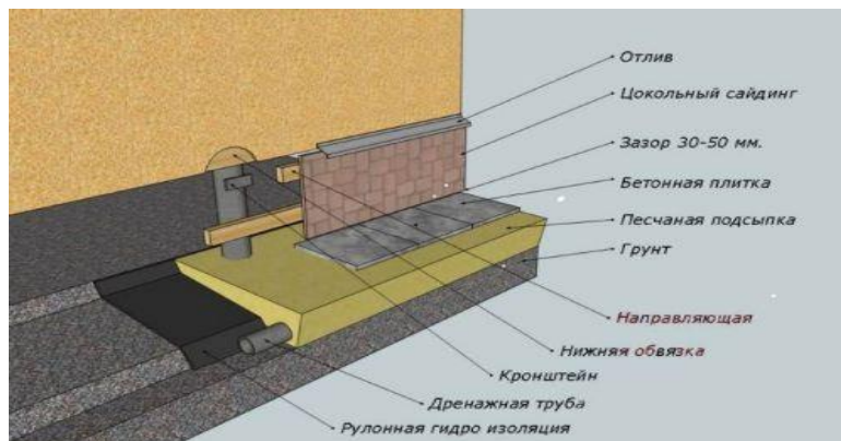
5-расм. Биноларнинг пойдевор конструкциялари билан жихозланган ва ер ости сувларини қочириш учун дренаж трубаларидан фойдаланилган курси ечими.
